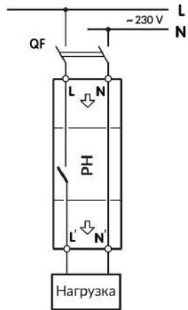
QF - двухполюсный автоматический выключатель
