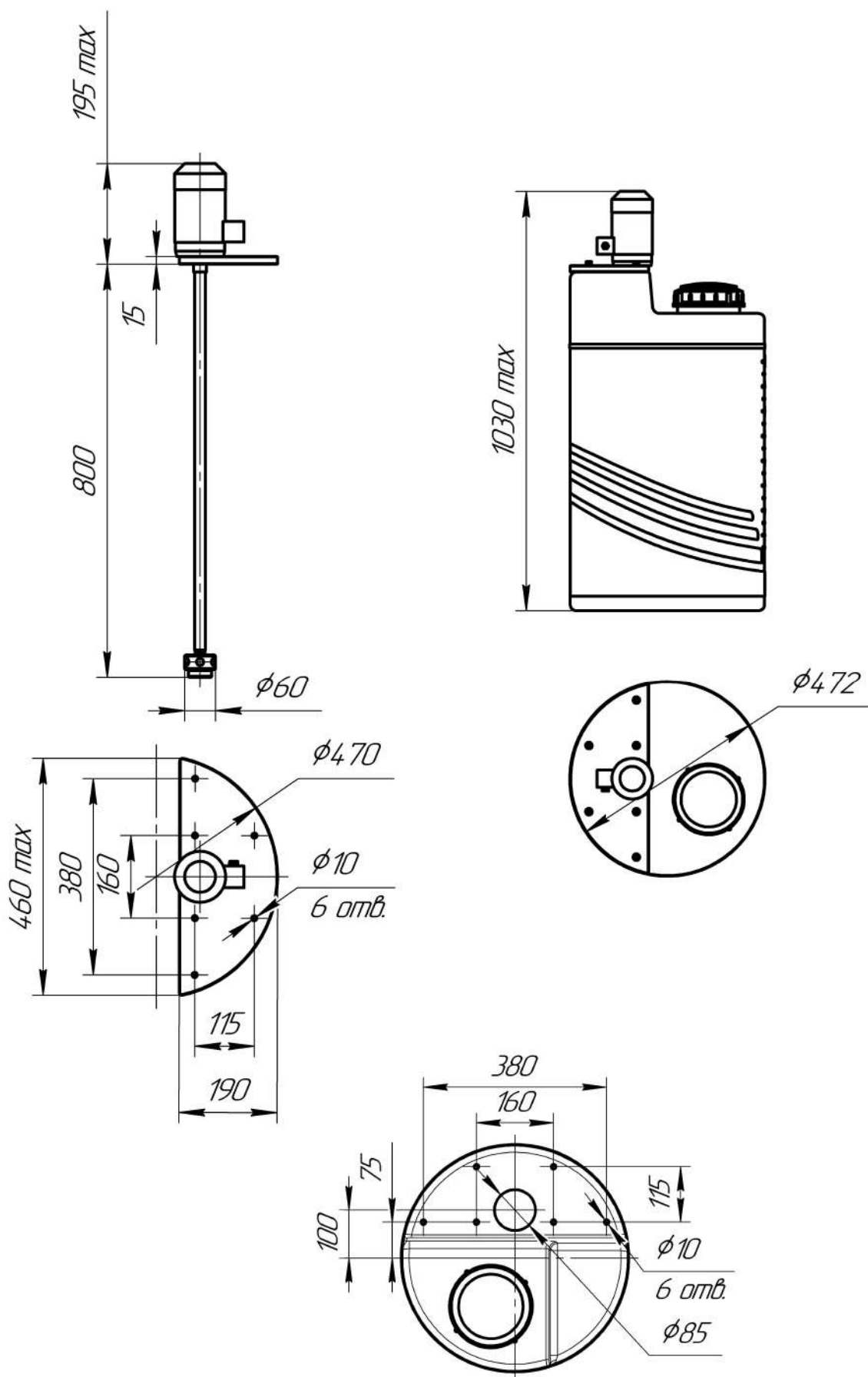
Габаритные размеры дозирочной ёмкости объёмом 100 литров с установленной мешалкой
