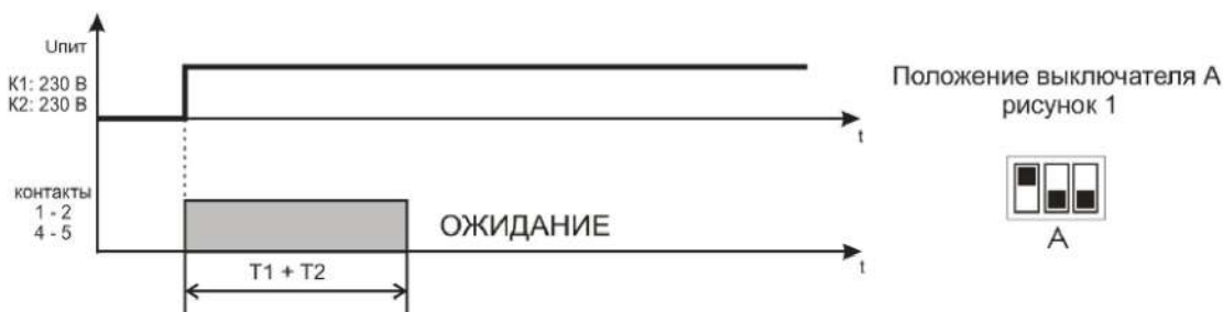
Рисунок 7 – Алгоритм работы Реле импульсное 2
