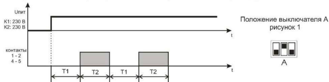
Рисунок 5 – Алгоритм работы Реле периодическое 1 (с задержкой на включение)
