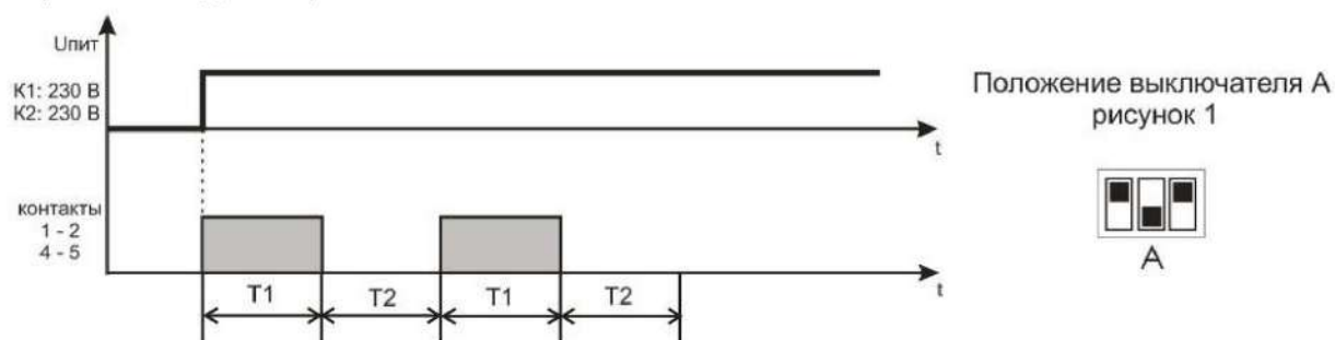
Рисунок 8 – Алгоритм работы Реле периодическое 2
