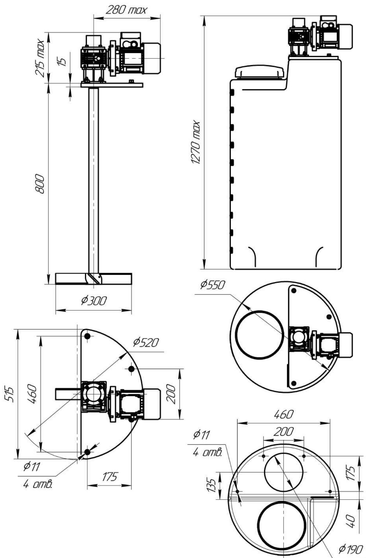
Габаритные размеры дозирующей ёмкости 200 литров с установленной мешалкой
