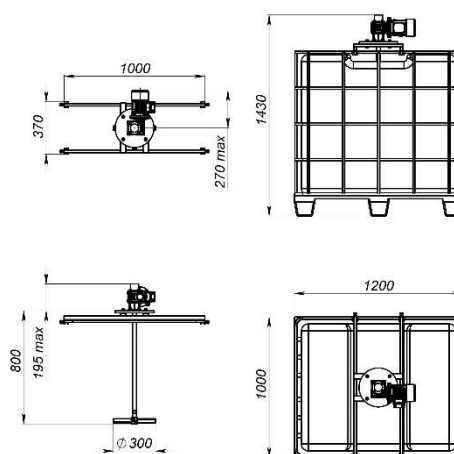
Габаритные размеры емкости "Еврокуб" с установленной мешалкой
