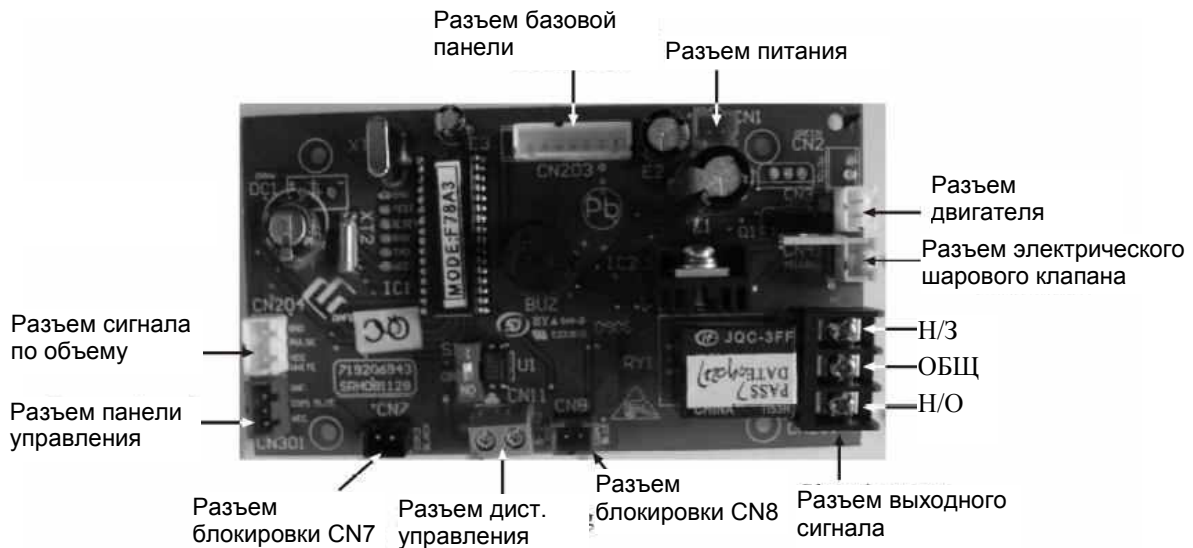
Рисунок 3: Главная плата управления
