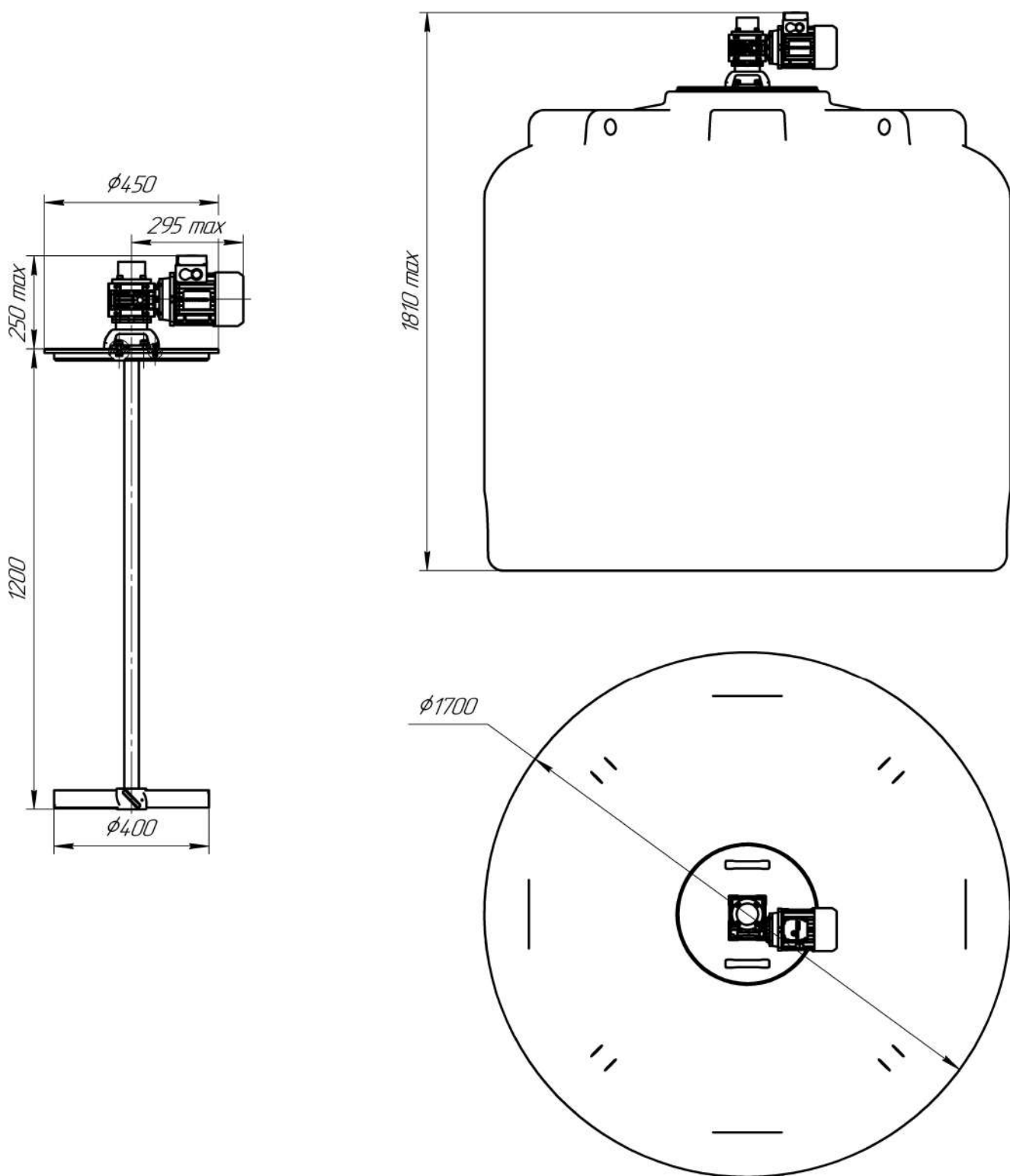
Габаритные размеры емкости TR 3000 с установленной мешалкой
