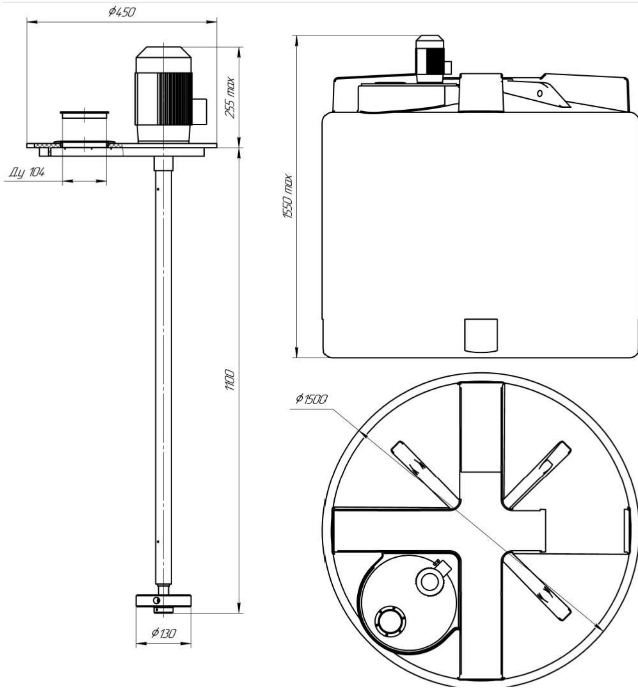
Габаритные размеры емкости Т 2000 с установленной мешалкой
