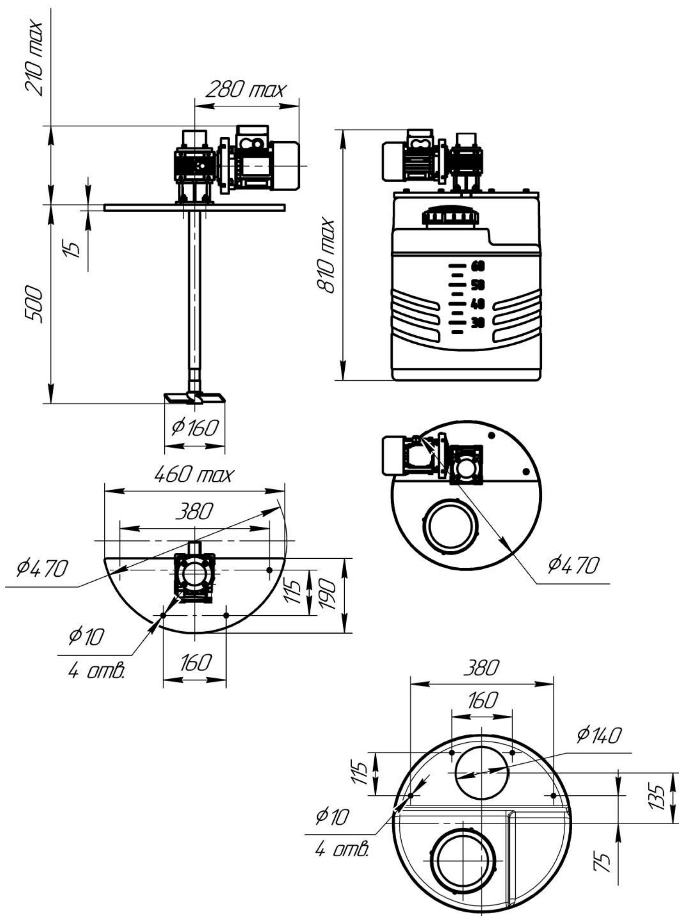
Габаритные размеры дозировочной ёмкости объёмом 60 литров с установленной мешалкой
