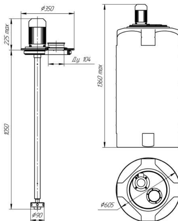
Габаритные размеры емкости Т 300 с установленной мешалкой
