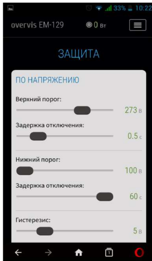
Рисунок А5 – Защита по напряжению
