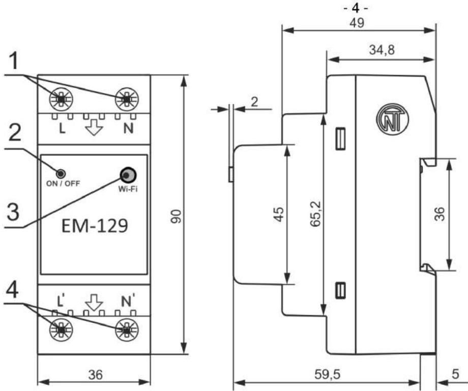
Рисунок 1 – Органы управления, габаритные и установочные размеры EM-129
