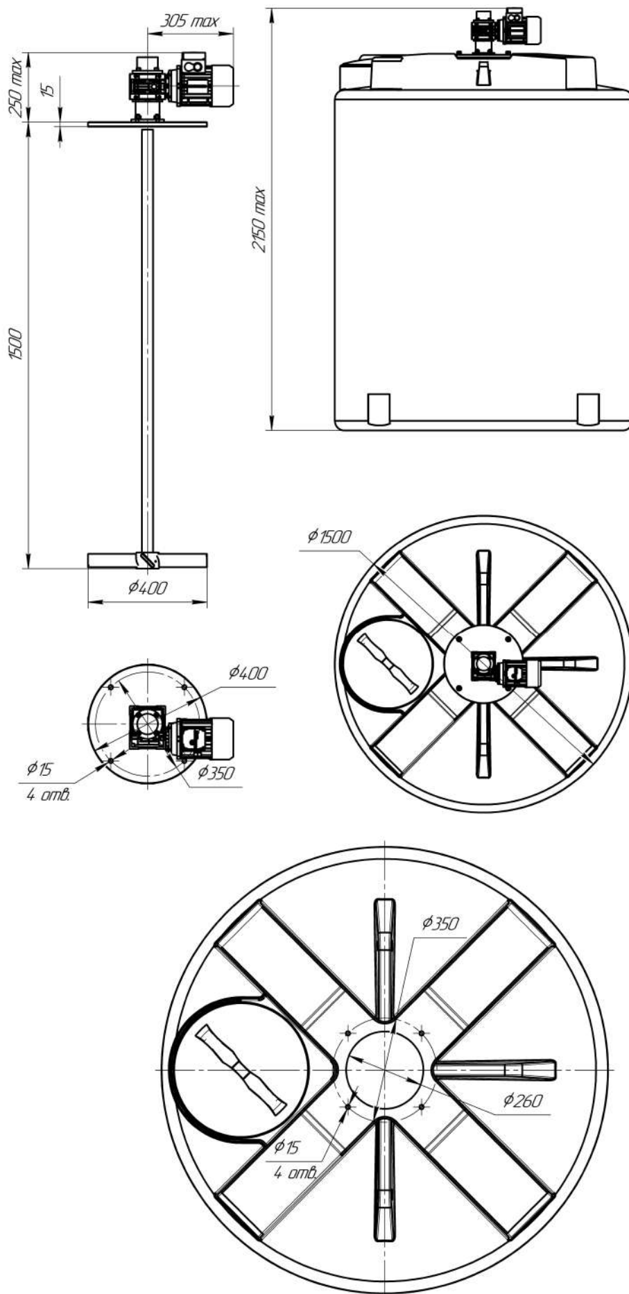
Габаритные размеры емкости Т3000 с установленной мешалкой
