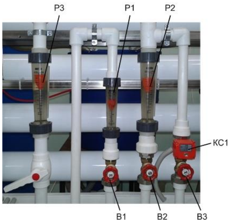
Рис.2 Ротаметры и вентили.
