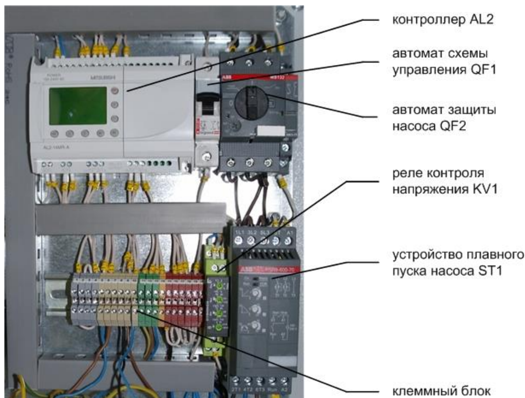
Рис.6 Блок управления – вид изнутри.
