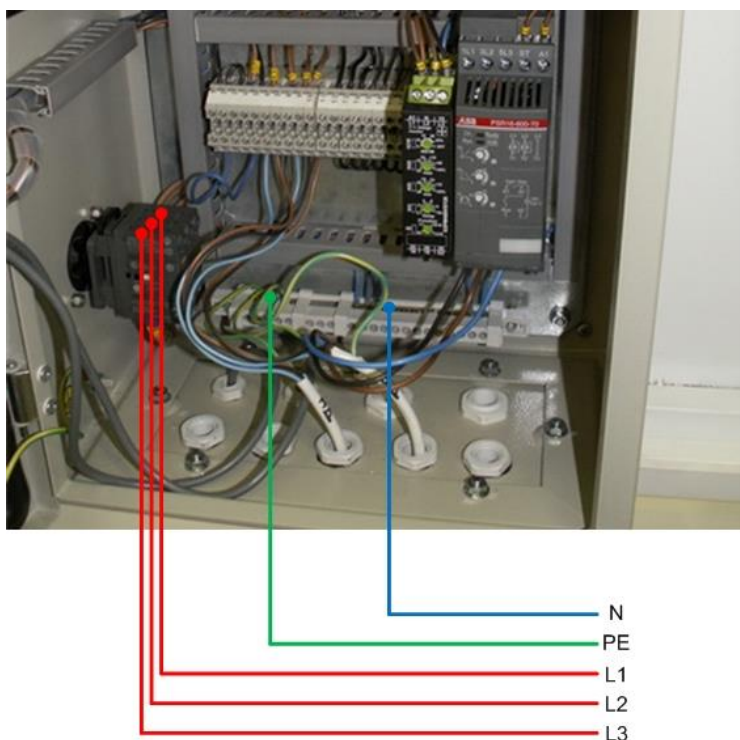
Рис.8 Подключение электропитания.
