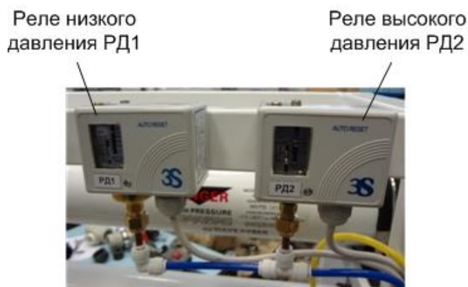
Рис.4 Реле давления.
