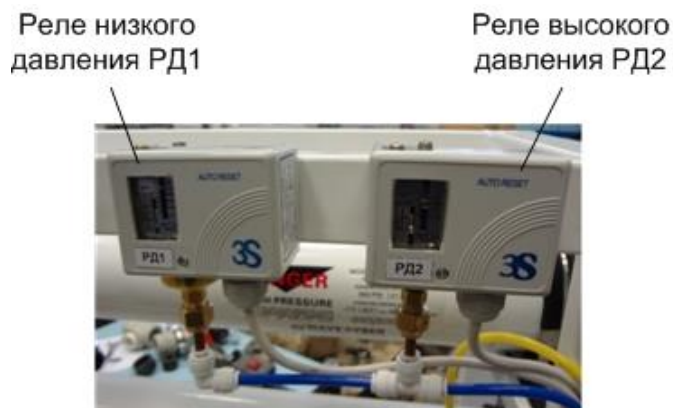
Рис.4 Реле давления.
