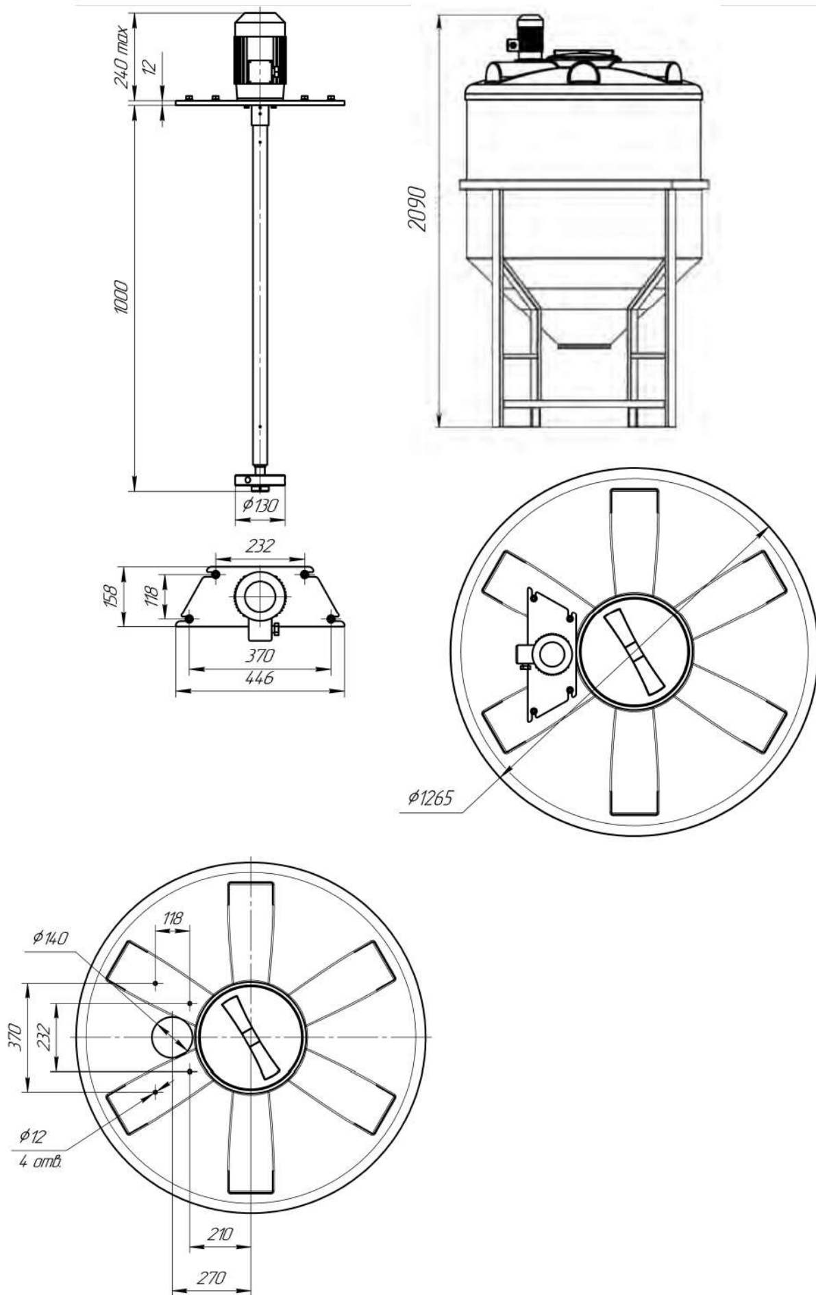
Габаритные размеры емкости ФМ 1000 с установленной мешалкой
